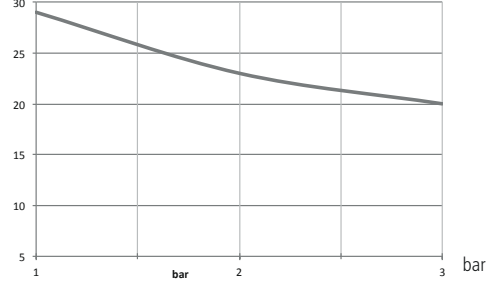
0320: l/h 20 bar 3 Corps de pompe mod. SA
