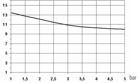
0320: l/h 20 bar 3 Corps de pompe mod. SA
