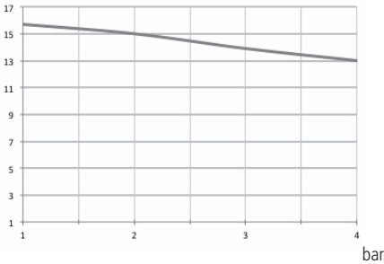
0135: l/h 35 bar 1 Corps de pompe mod. TA
