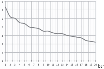
0413: l/h 13 bar 4 Corps de pompe mod. NA
