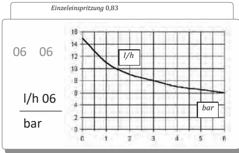
Einzeleinspritzung 0,83
